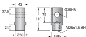
Clevis End (optional): 9001-EM-02
