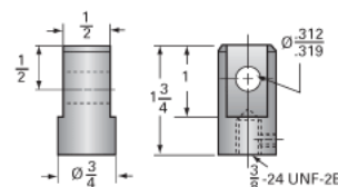
Clevis End (optional): 9001-00-12
