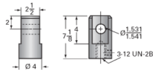
Clevis End (optional): 9001-00-16
