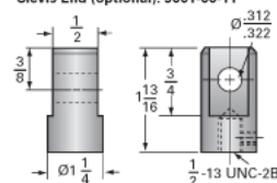
Clevis End (optional): 9001-00-11
