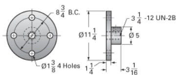
Top Plate (optional): 9000-00-09
