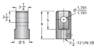
Clevis End (optional): 9001-00-09
