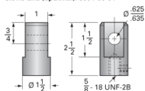
Clevis End (optional): 9001-00-01
