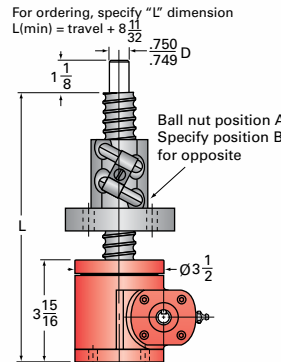
3-BSJ-UR UPRIGHT ROTATING
