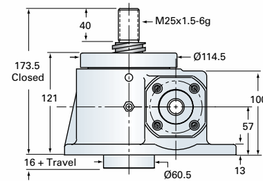
EM5-MSJ-U UPRIGHT
