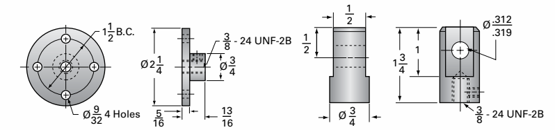
MINI CUBIC JACK Options (Standard Steel Parts)
