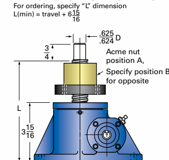
2R-MSJ-UR UPRIGHT ROTATING
