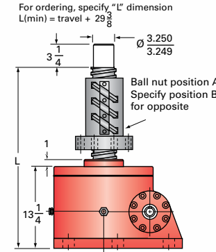
100-BSJ-UR UPRIGHT ROTATING
