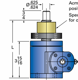
2-MSJ-UR UPRIGHT ROTATING
