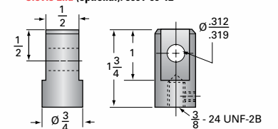
Clevis End (optional): 9001-00-12
