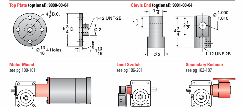
10-BSJ & 10HL-BSJ Options
