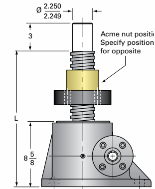
25SS-MSJ-UR UPRIGHT ROTATING
