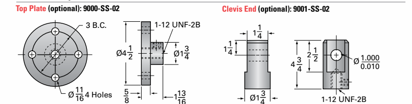
5SS-MSJ Options
