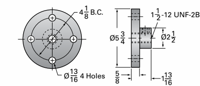
15SS-MSJ Options
