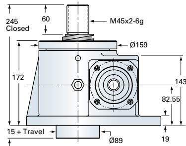
EM20-MSJ-U UPRIGHT
