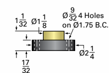
MINI JACK Acme Nut and Flange
