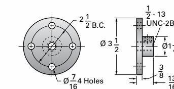
1-BSJ Options
