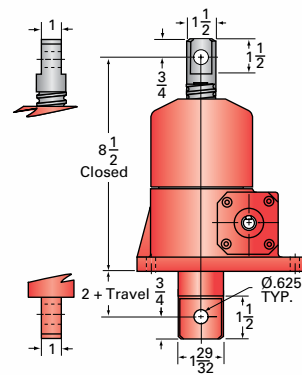
2.5HL-BSJ DOUBLE CLEVIS
