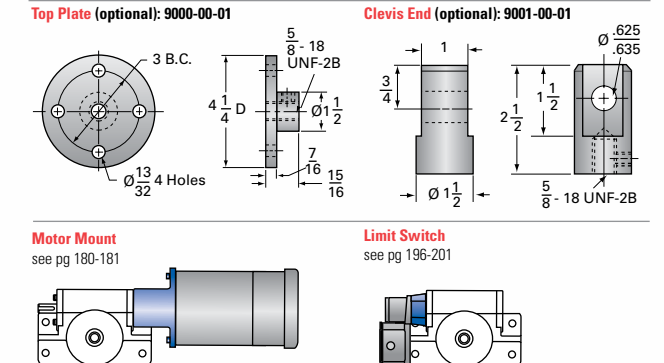
2-MSJ Options
