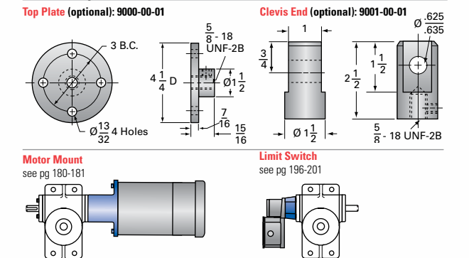
2R-MSJ Options
