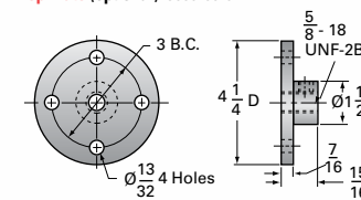
3-BSJ Options
