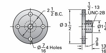
1HL-BSJ Options
