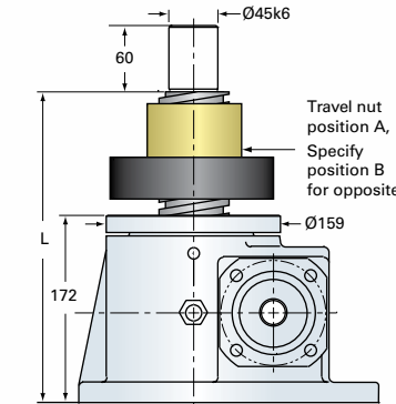
EM20-MSJ-UR UPRIGHT ROTATING
