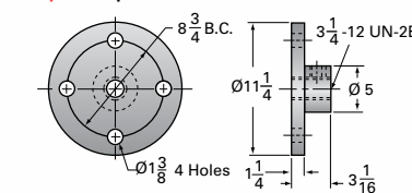
50-MSJ Options
