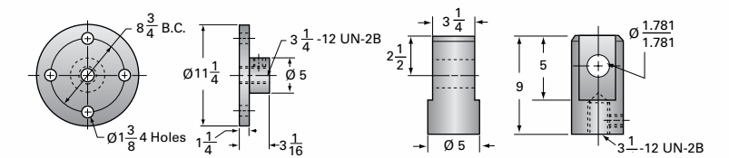
50-BSJ Options
