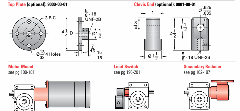
2.5HL-BSJ Options
