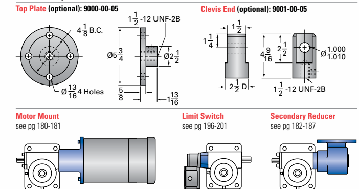
15-MSJ Options
