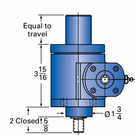
2-MSJ-I INVERTED
