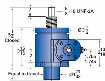
2-MSJ-U UPRIGHT
