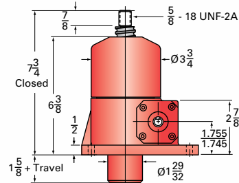
2.5HL-BSJ-U UPRIGHT
