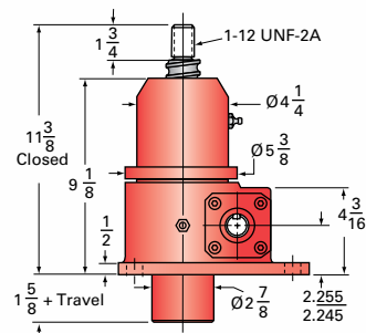
10-BSJ-U & 10HL-BSJ-U UPRIGHT
