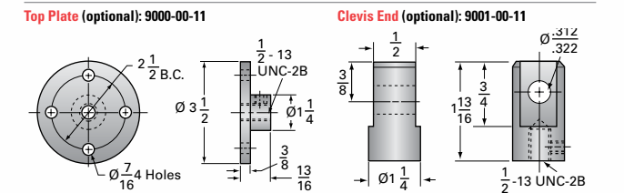
1-MSJ Options
